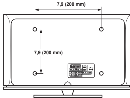
VISTA POSTERIOR
